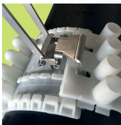
Applicazione di un collare F.
